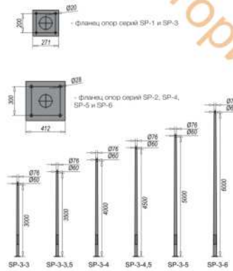
Размеры фланцев опор:
